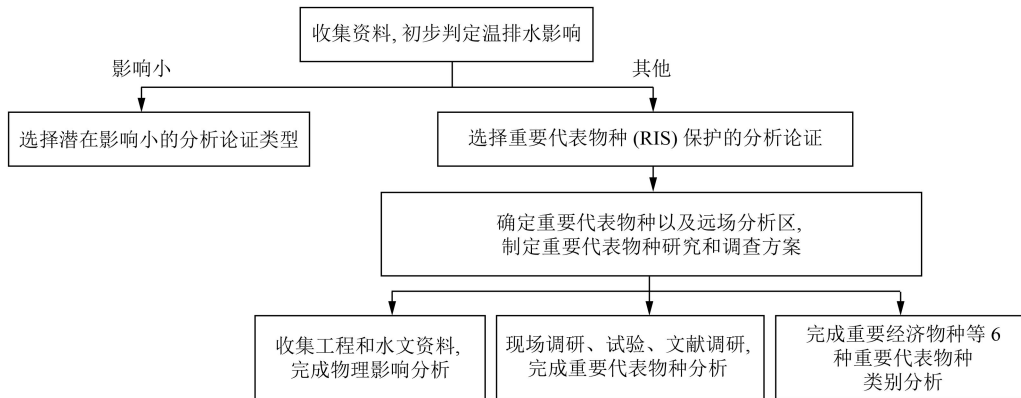
图 3 核电厂建造阶段温排水环评分析论证流程
