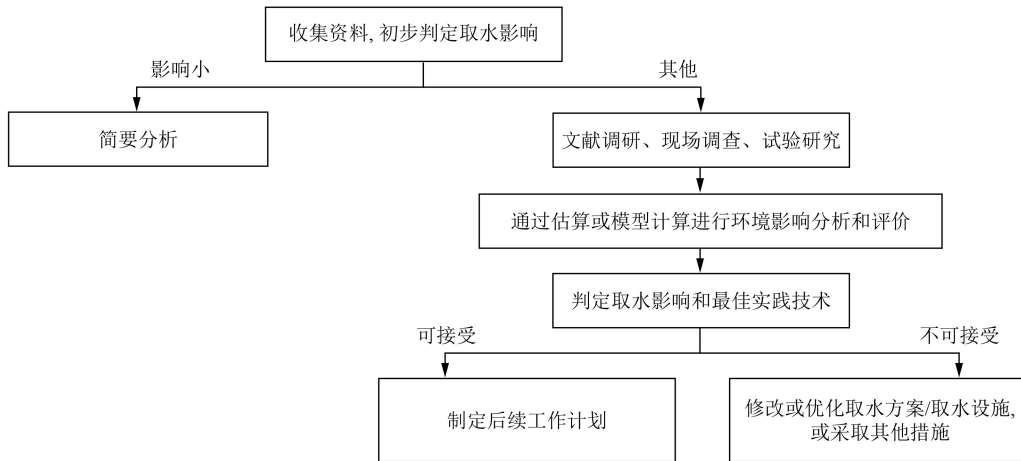
图 2 核电厂建造阶段取水环评分析论证流程
