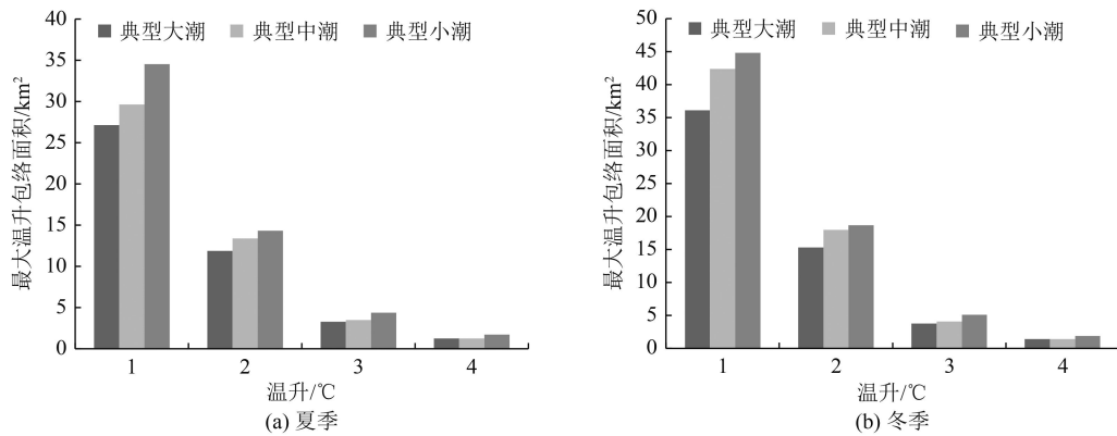
图 1 北方某核电厂夏季、冬季 6 台机组运行期间各典型潮条件下温升包络面积
